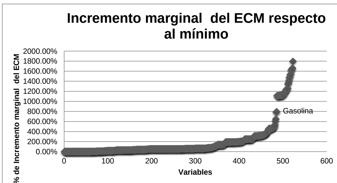
Figura 5. Incrementó del ECM para cada una de las 524 variables
