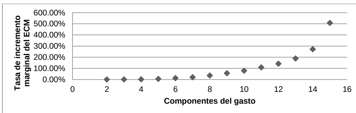
Figura 4. Tasas de incremento marginal del ECM respecto al mínimo obtenido
