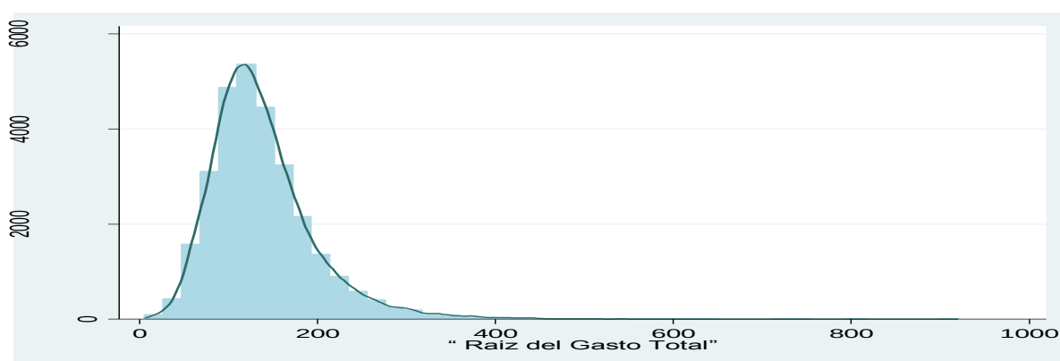
Figura 2. Distribución y frecuencia de la raíz del gasto corriente monetario
