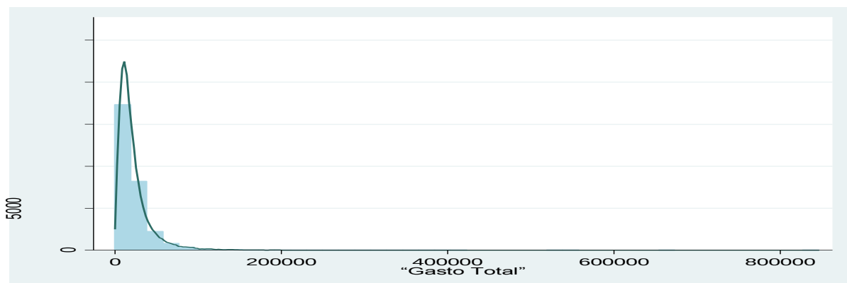
Figura 1. Distribución y frecuencia del gasto corriente monetario
