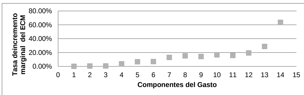
Figura 3. Tasas de incremento marginal del ECM
